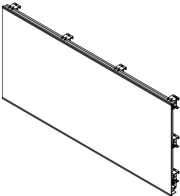
Кассета с тонкой керамогранитной плитой и креплением на аграфы: горизонтальные поддерживающие и вертикальные фиксирующие планки
