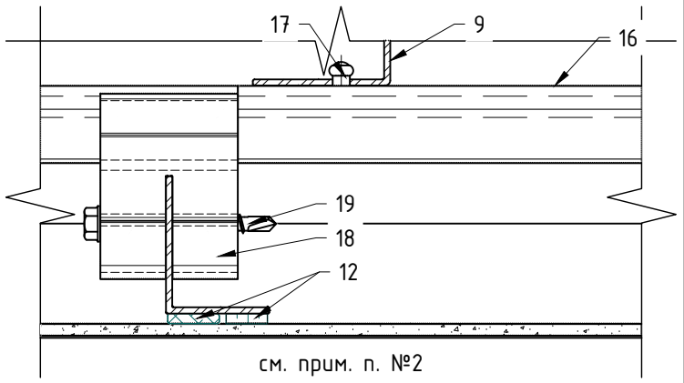
Фрагмент №1 (вариант с вертикальными несущими и горизонтальными поддерживающими профилями, положение направляющей в середине аграфного профиля)
