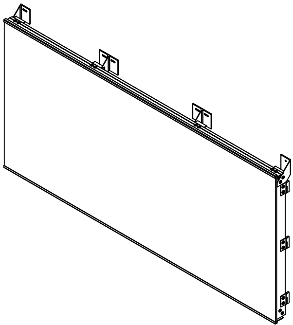
Кассета с тонкой керамогранитной плитой и креплением на салазки: горизонтальные поддерживающие и вертикальные фиксирующие планки
