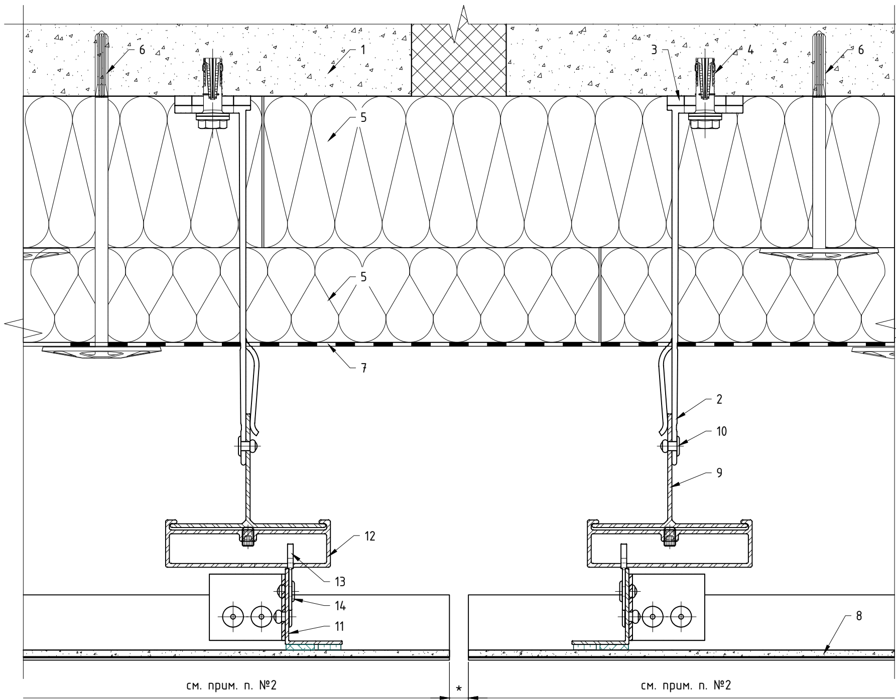
7.10. Деформационный шов: элементы "Light", скрытое крепление на салазки.
