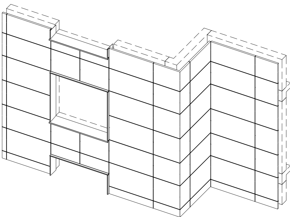
Кассета из тонкого керамогранита: крепление на салазки или аграфы, горизонтальное положение облицовки
