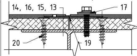
Сечение А-А (вар. 3)
