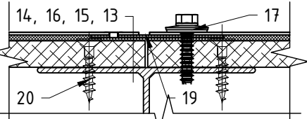
Сечение А-А (вар. 3)
