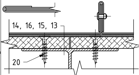
Сечение Б-Б
