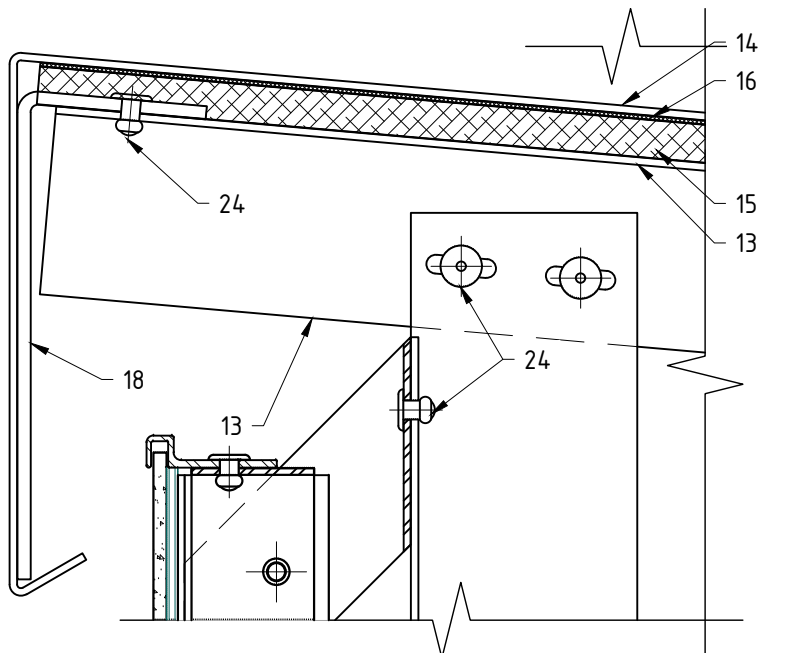
Вариант крепления парпетной крышки №3
