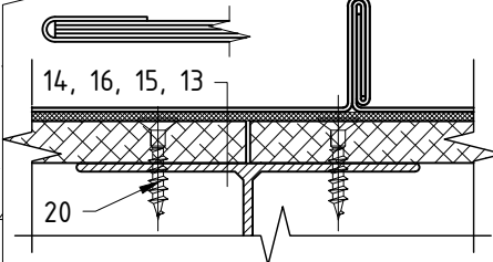
Сечение Б-Б
