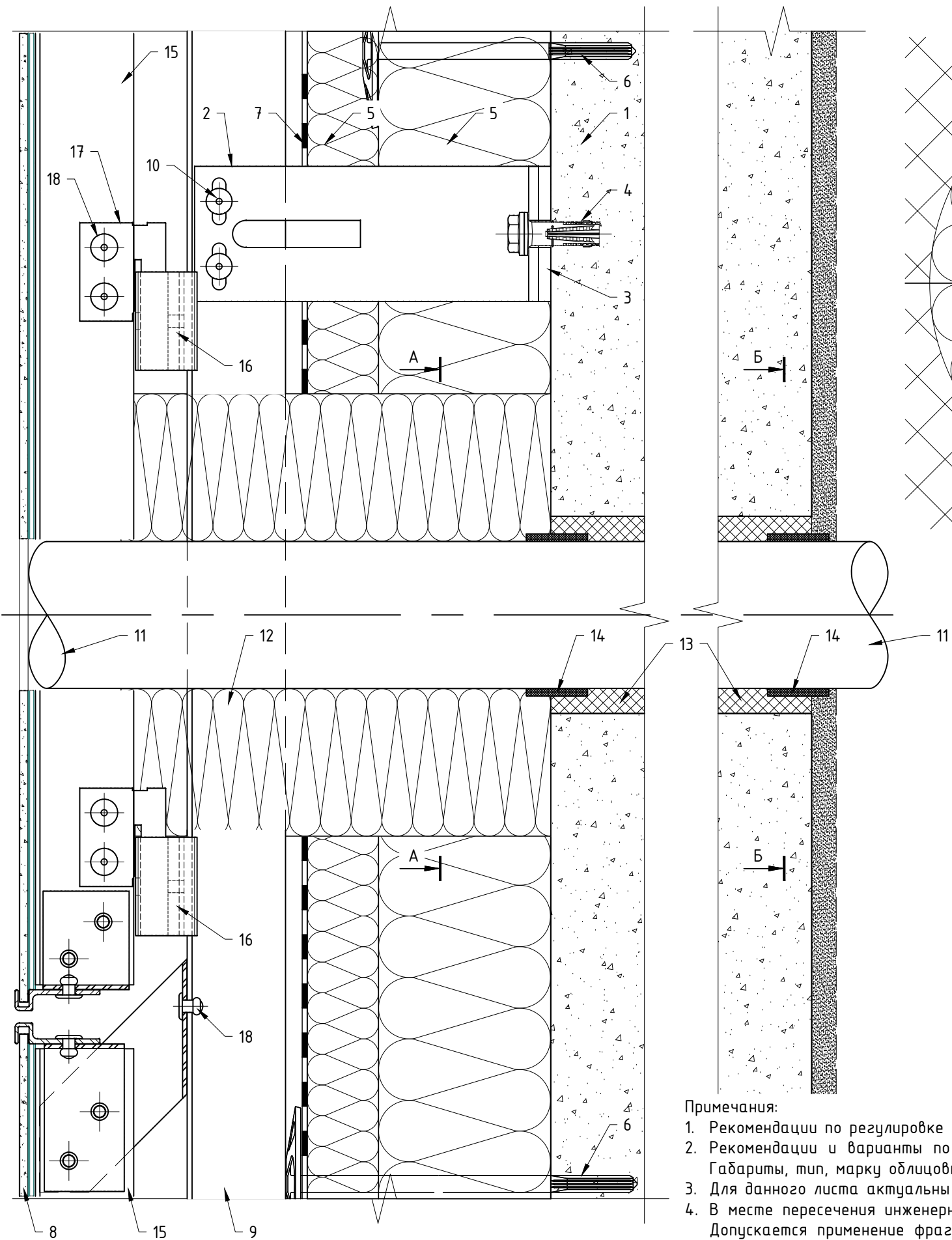
7.11. Ввод коммуникаций: элементы "Light", скрытое крепление на салазки.
