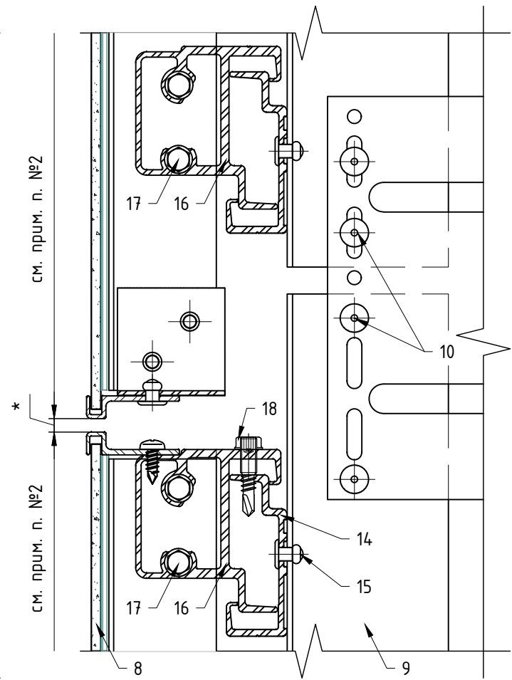
Фрагмент №1 (вариант с креплением на анграфы)
