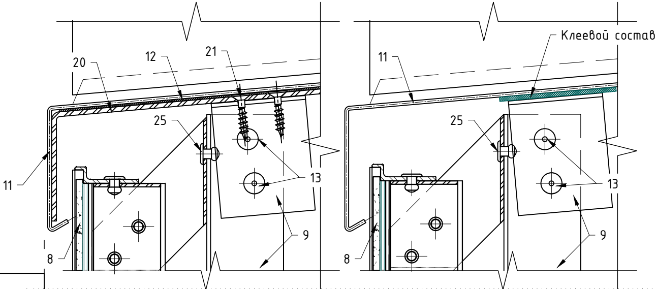
Фрагмент №1: доп. варианты крепления отлива к направляющей
