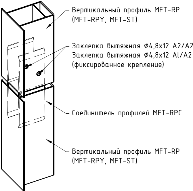
Узел №6 (увеличено)
