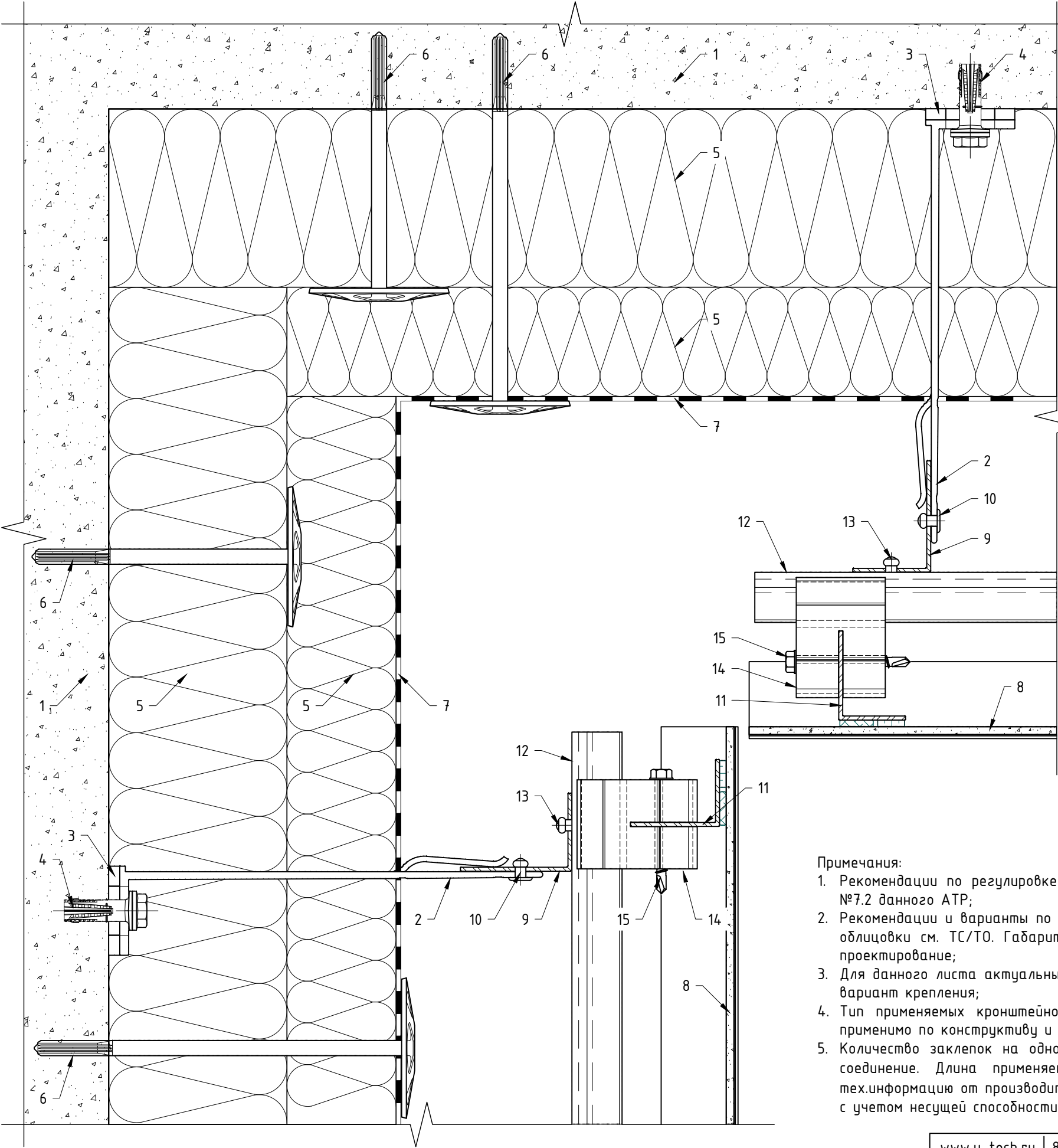
Выполнение внутреннего угла фасада: вариант №1, элементы "Light", скрытое крепление на аграры.
