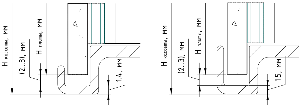
Узел №1 (увеличено)
