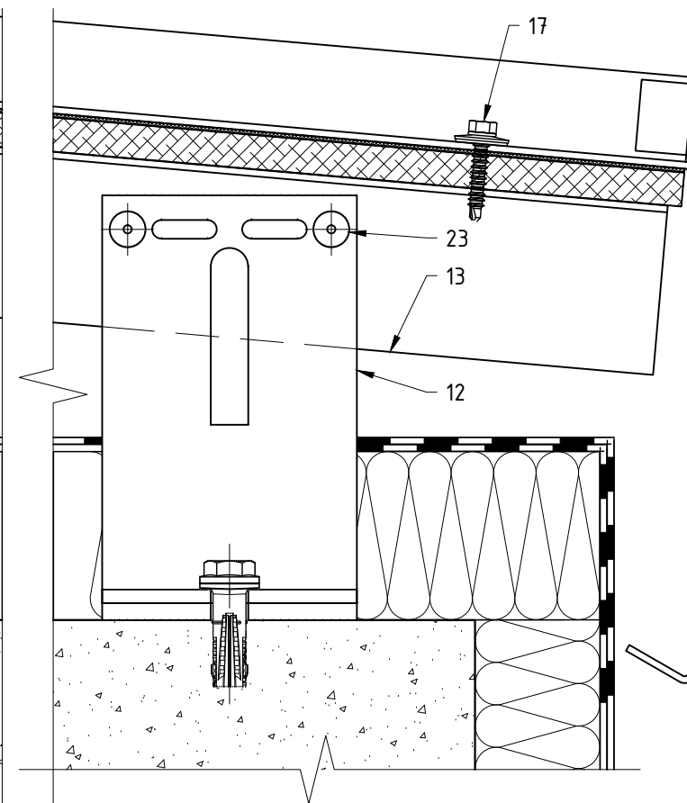
Сечение А-А (вар. 1, вар.2)
