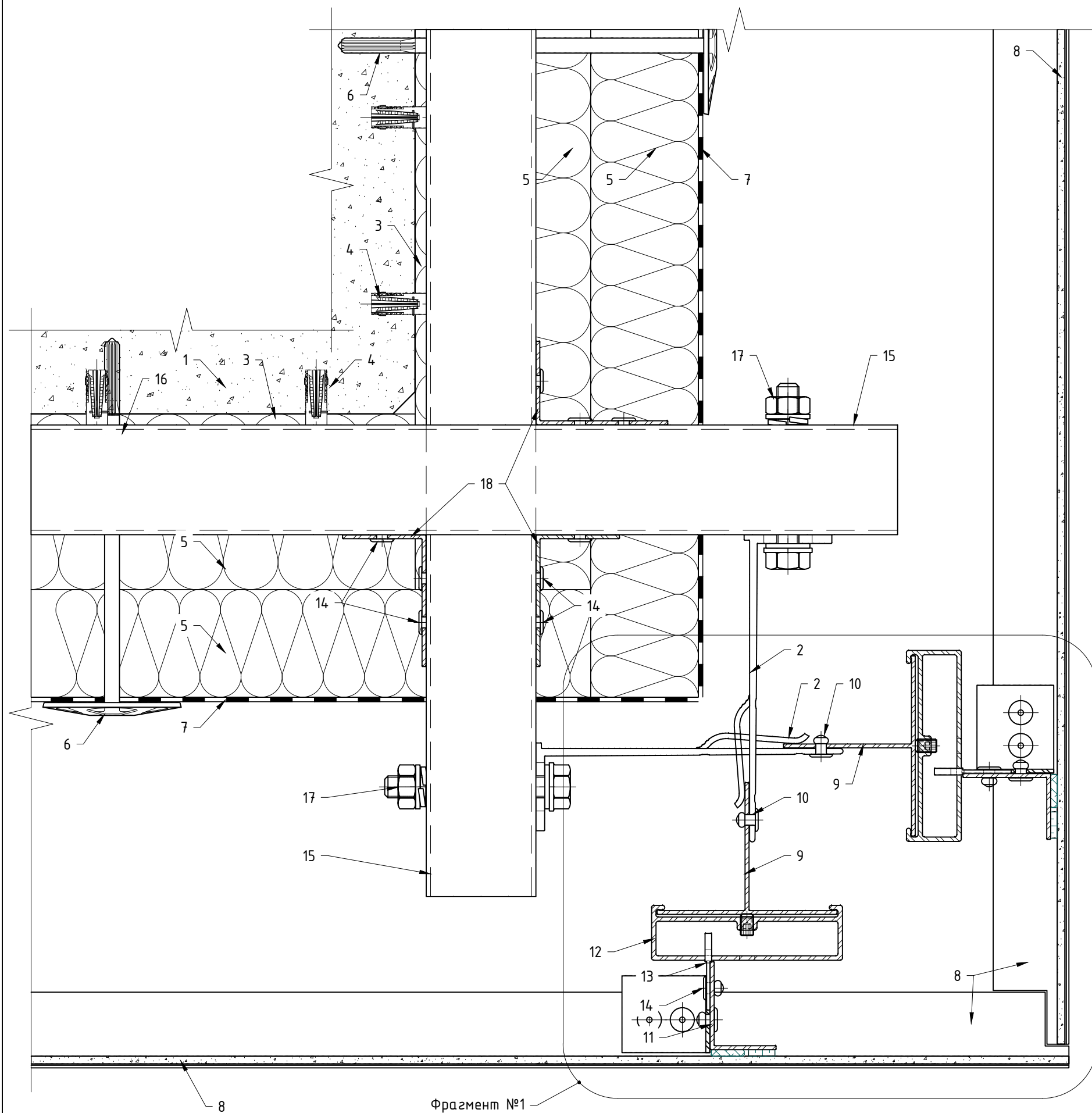
7.7. Выполнение наружного угла фасада: элементы "Light", скрытое крепление на салазки, вариант №1.
