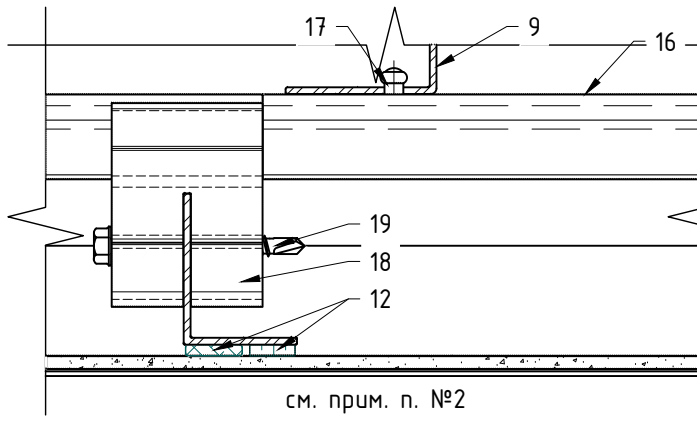
Фрагмент №1 (вариант с горизонтальными несущими профилями, положение направляющей в середине аграфного профиля)
