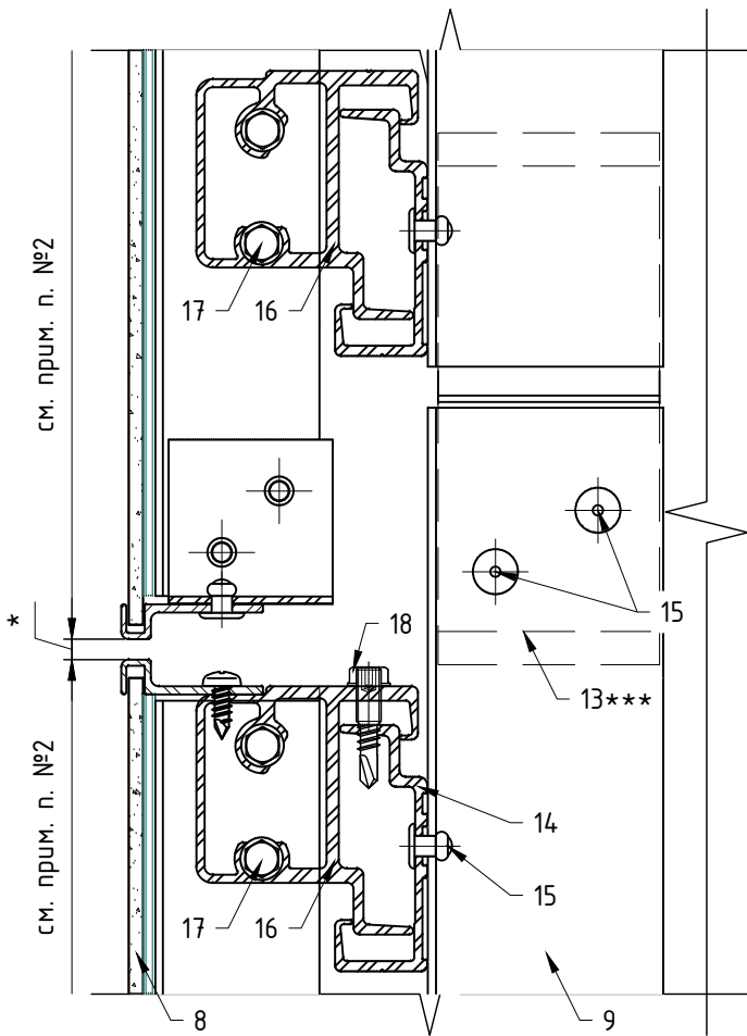
Фрагмент №1 (вариант с креплением на аграфы)
