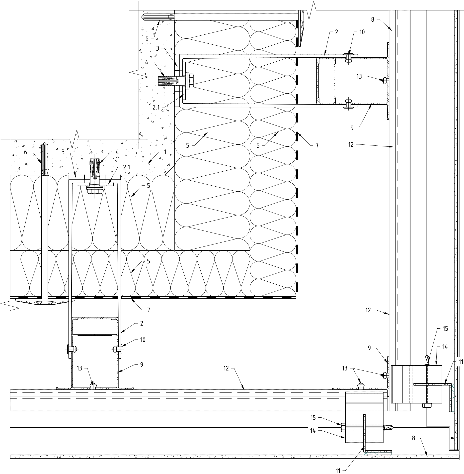
Выполнение наружного угла фасада: элементы "Heavy", скрытое крепление на анграфы, вариант №2.
