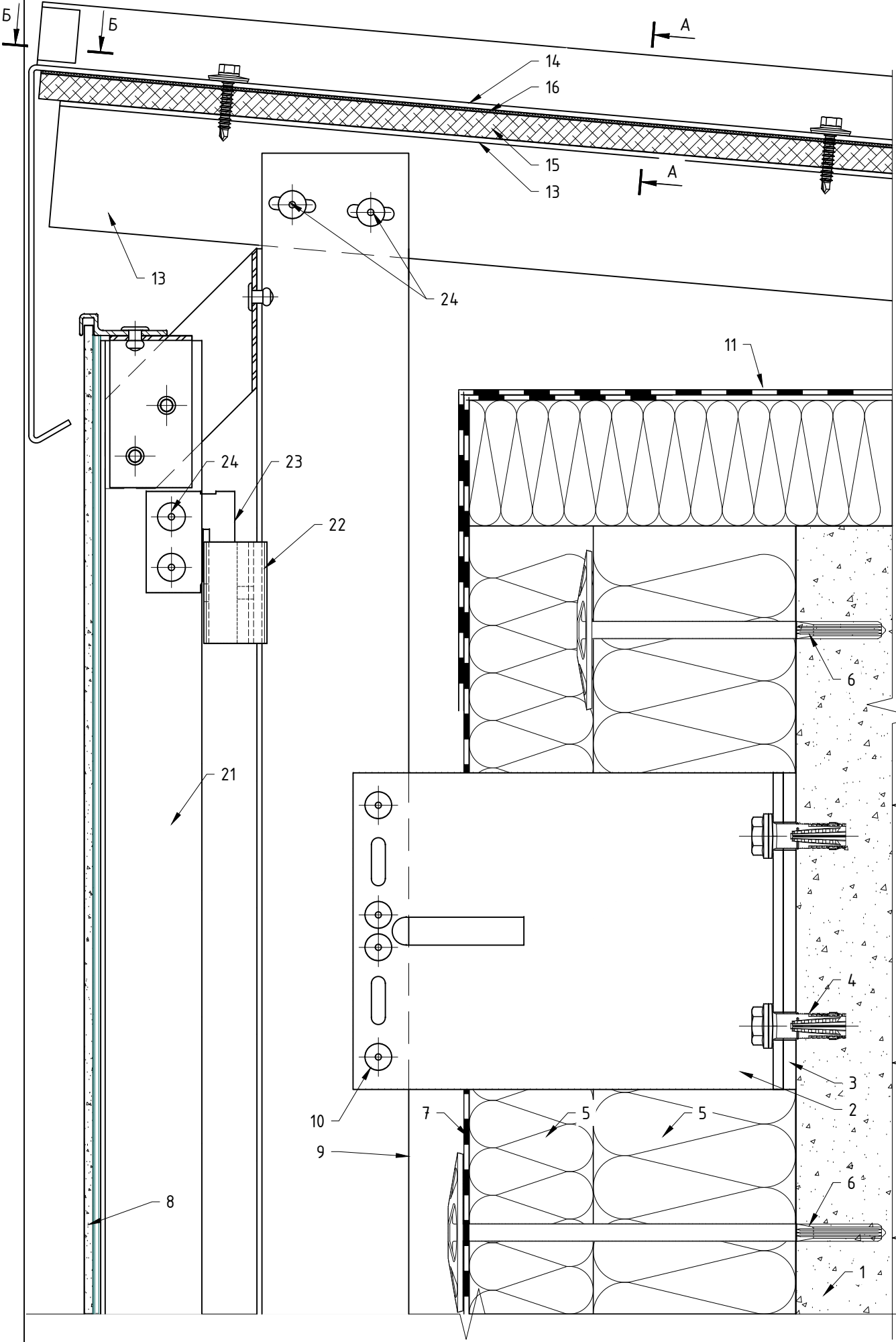
7.9. Примыкание к парапету: вариант крепления парпетной крышки №1, элементы "Light", скрытое крепление на салазки.
