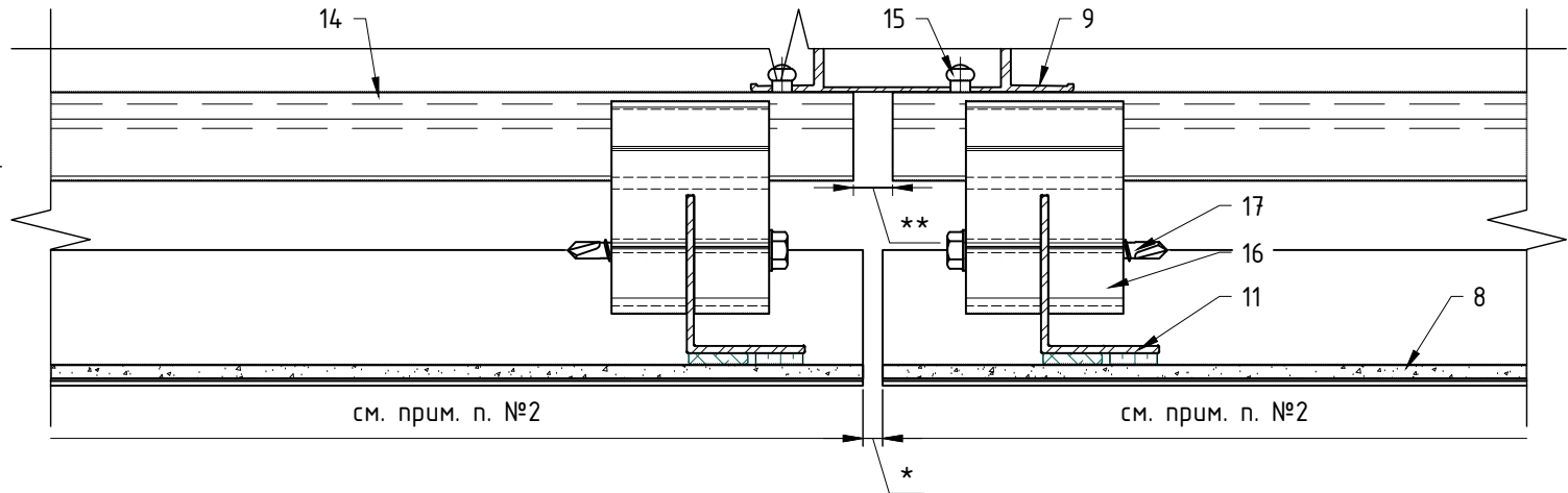
Фрагмент №1 (вариант крепления на аграфах)
